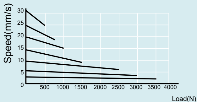
速度-负载图
