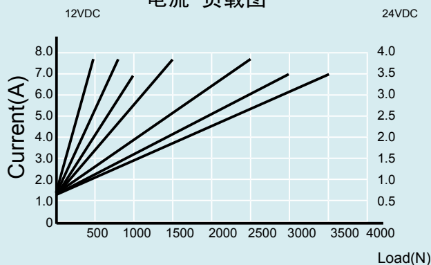
电流-负载图
